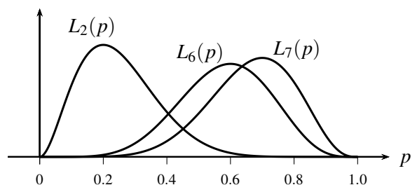
Abb. 10: Likelihoodfunktionen ( n = 10 )
